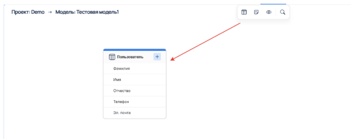
Рисунок 25 - Создание таблицы
